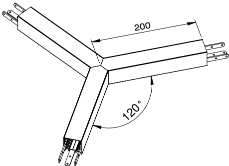
3-Way Y Scale 1:7
